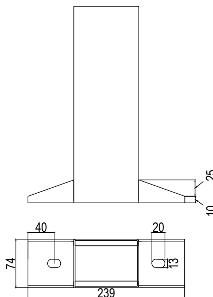
RiSySchott-Stütze 75
