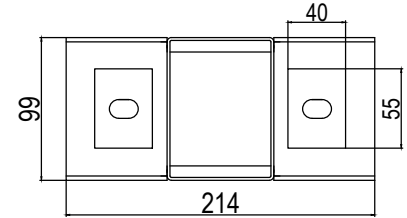
RiSySchott-Stütze 100
