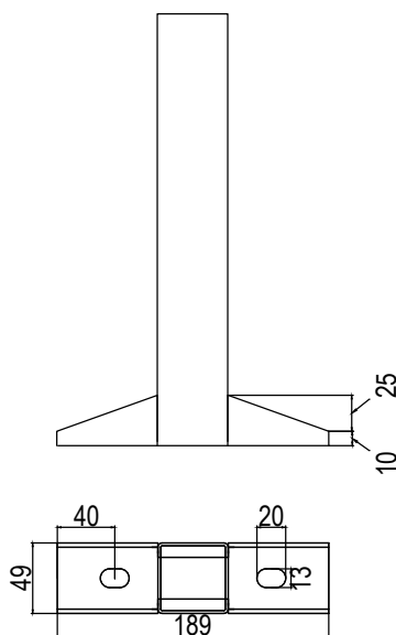
RiSySchott-Stütze 50
